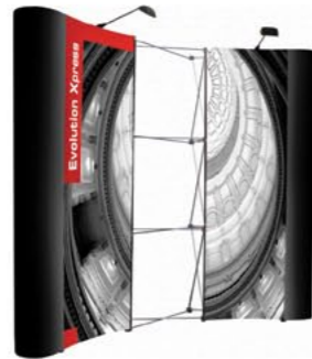
Ultima Evolution Xpress 3x3 Grafika teljes mérete: 2225x3365mm A PopUp fal szélessége felállítva 2540mm Grafikai panelek: Front panel: 3db 2225mmx673mm Oldalsó panel: 2db 2225x673mm
